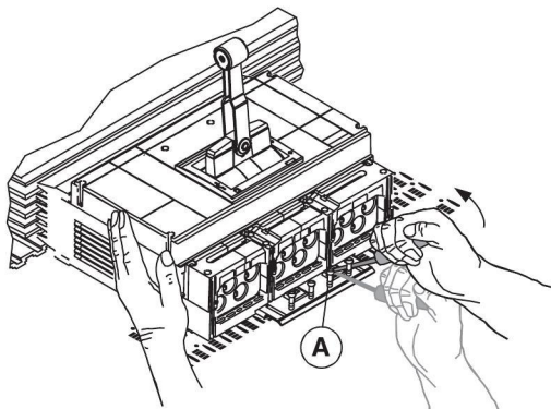
Figura 6: Inserción del interruptor automático en la barra
